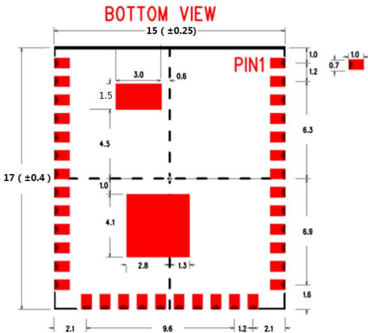
图 8-2. TX-AH-Rx00Pxx模组Bottom View
