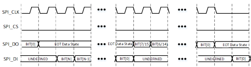
图 3-9: Microwire 格式的多收发时序
